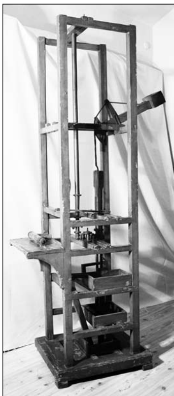
Модель венгерской водостолбовой машины. Автор П. Г. Ярославцев. 1823 г. Фонд Алтайского государственного краеведческого музея.
