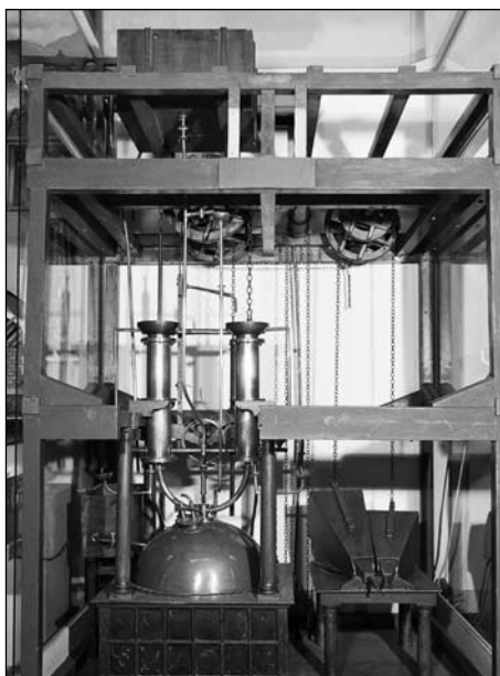
Модель пароатмосферной машины И. И. Ползунова по проекту 1763 г. Авторы П. Г. Ярославцев и И. С. Климов. 1825 г.
